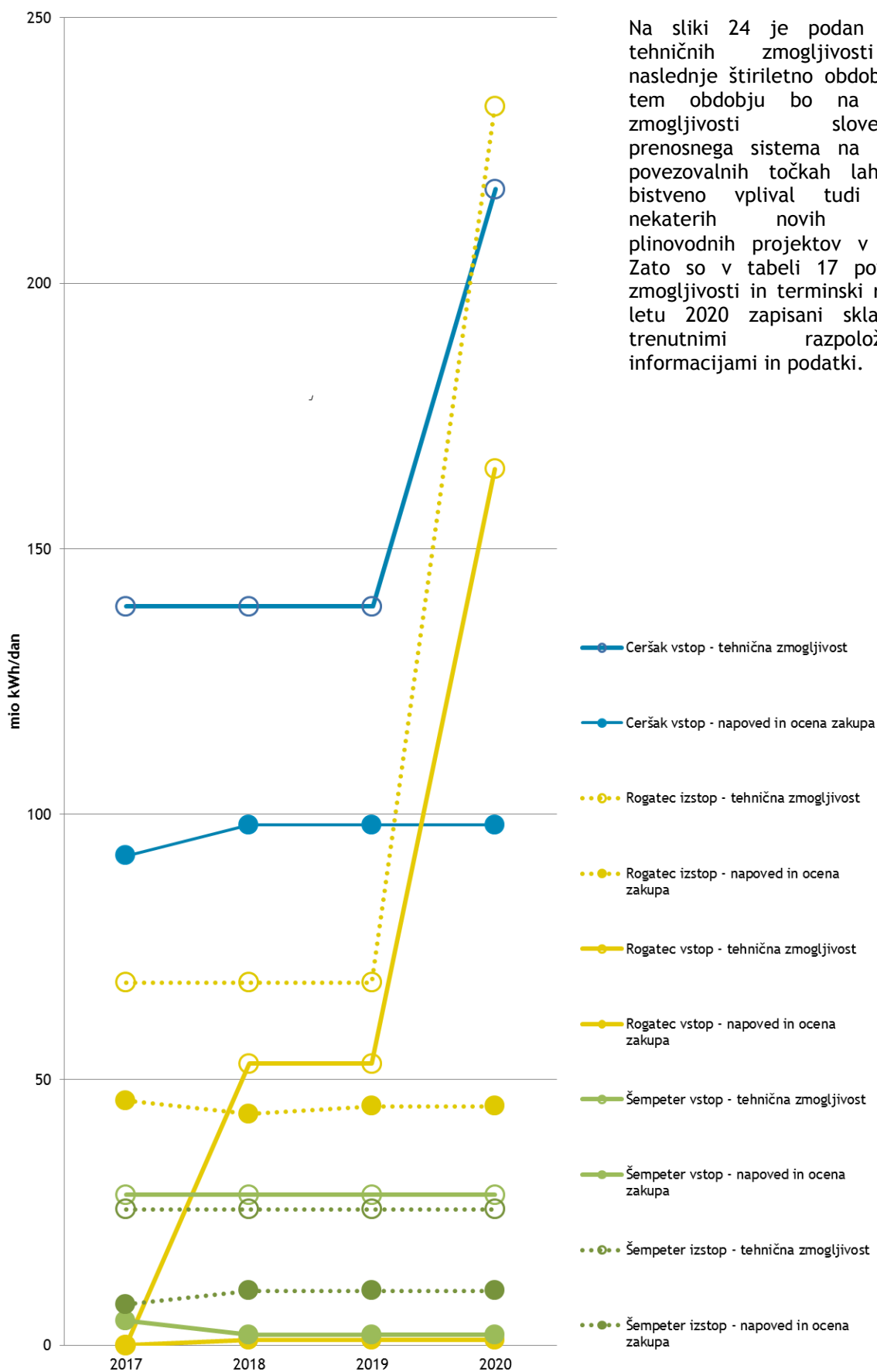
Slika 24. Tehnične zmogljivosti, napoved in ocena zakupa na povezovalnih točkah
