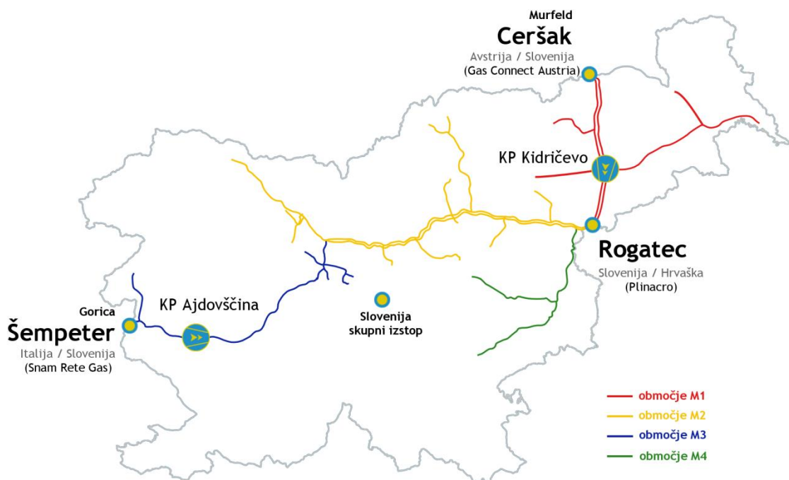
Slika 3. Shematski prikaz prenosnega plinovodnega sistema z relevantnimi točkami
