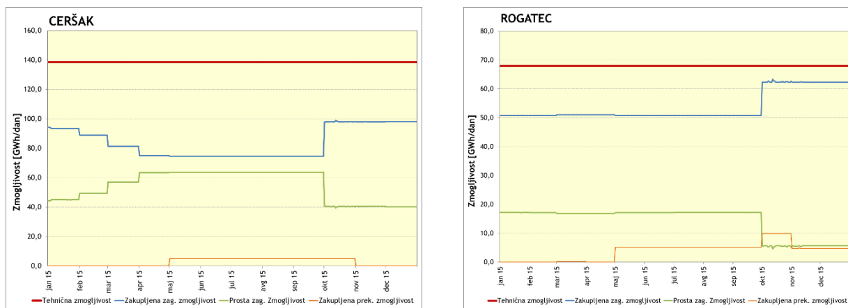
Slika 21. Prenosne zmogljivosti na mejnih povezovalnih točkah Ceršak in Rogatec v letu 2015
