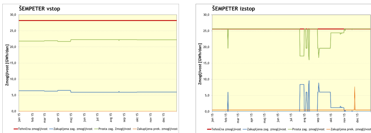
Slika 22. Prenosne zmogljivosti na mejni povezovalni točki Šempeter letu 2015
