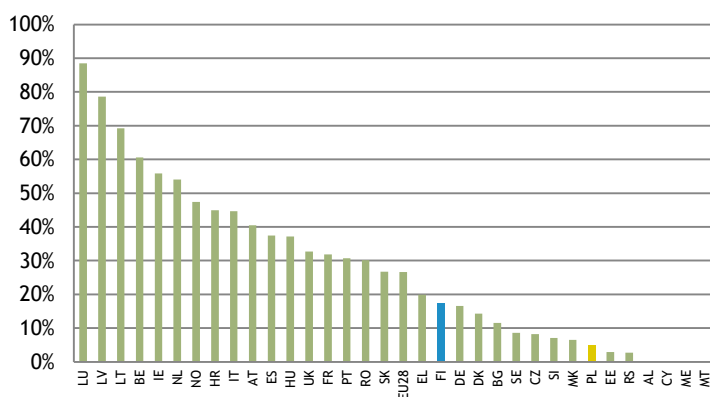
Slika 15. Delež zemeljskega plina med energetske viri v konvencionalnih elektrarnah (podatki za leto 2013, osveženi v 2015)
