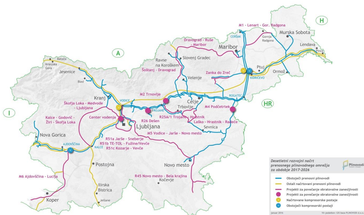
Slika 25. Lokacije projektov za povečanje obratovalne zanesljivosti
