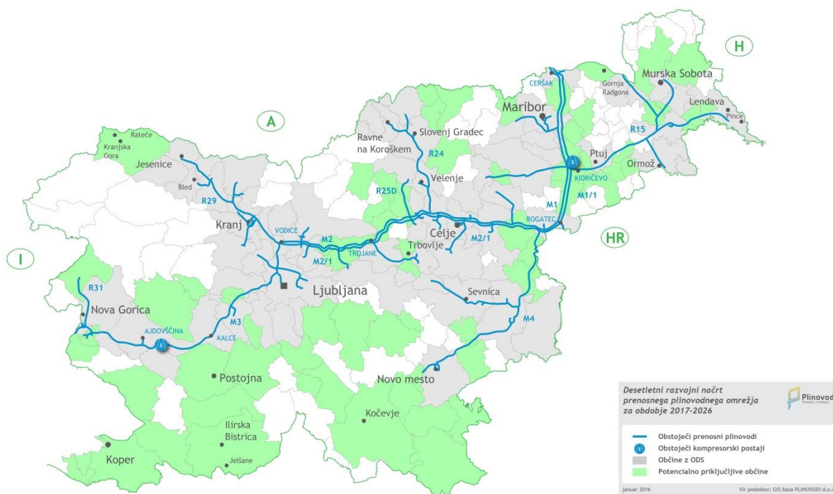
Slika 5. Regionalna razpoložljivost prenosnega plinovodnega sistema
