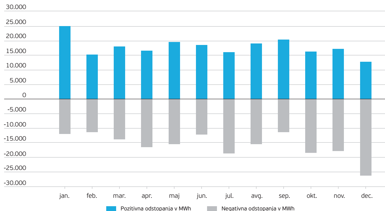
Slika 44: Mesečna odstopanja slovenskega omrežja v letu 2008
