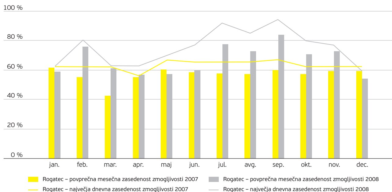
Slika 53: Največje dnevne in povprečne mesečne zasedenosti zmogljivosti merilno-regulacijske postaje Rogatec
