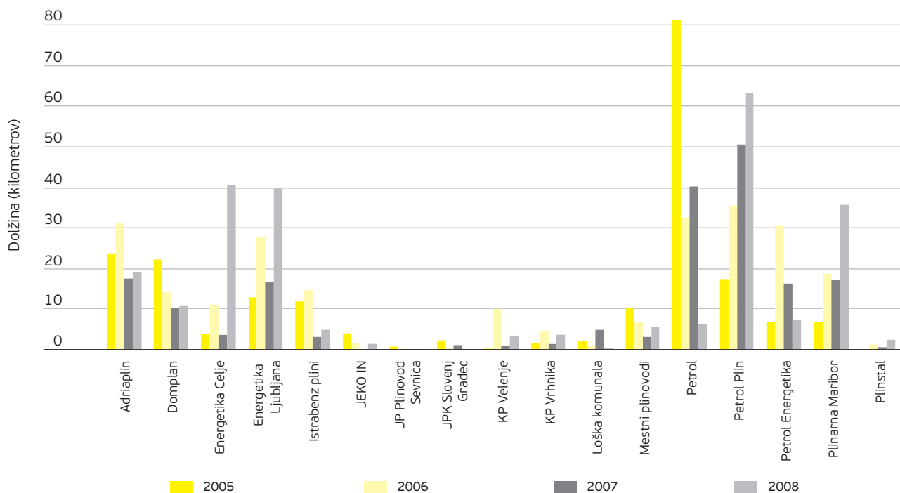
Slika 48: Dolžina novih distribucijskih omrežij v letih 2005–2008
