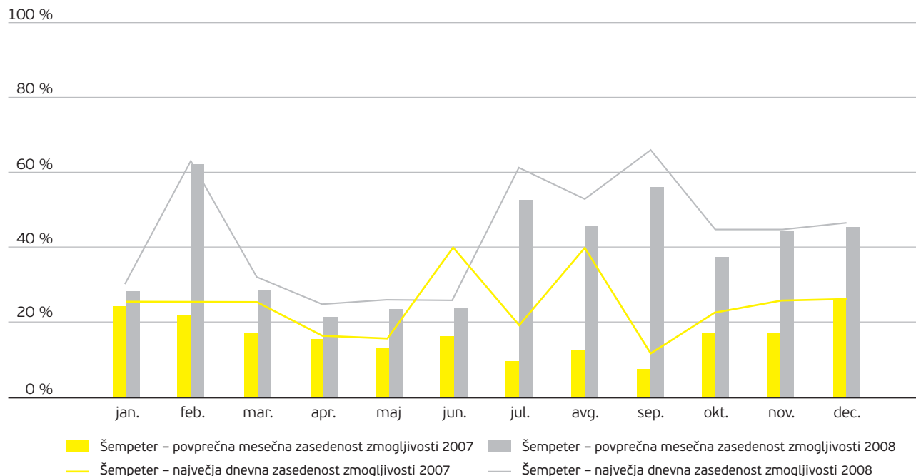
Slika 52: Največje dnevne in povprečne mesečne zasedenosti zmogljivosti merilno-regulacijske postaje Šempeter
