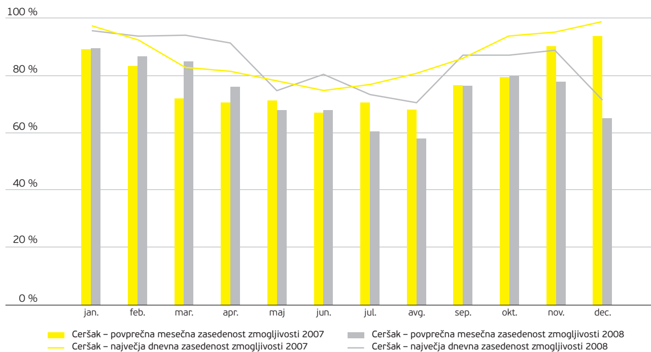
Slika 51: Največje dnevne in povprečne mesečne zasedenosti zmogljivosti merilno-regulacijske postaje Ceršak
