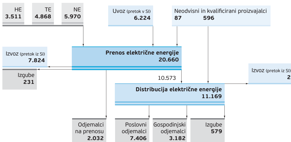
Slika 1: Elektroenergetska bilanca proizvodnje in porabe električne energije v letu 2008 v GWh
