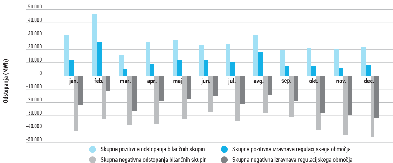
Slika 7: Skupna odstopanja v slovenskem elektroenergetskem sistemu v letu 2012
