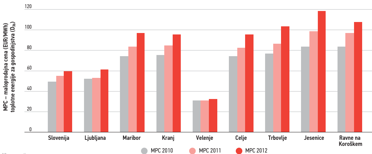
Slika 78: Gibanja povprečne maloprodajne cene daljinske toplote za gospodinske odjemalce v posameznih slovenskih mestih v obdobju 2010–2012
