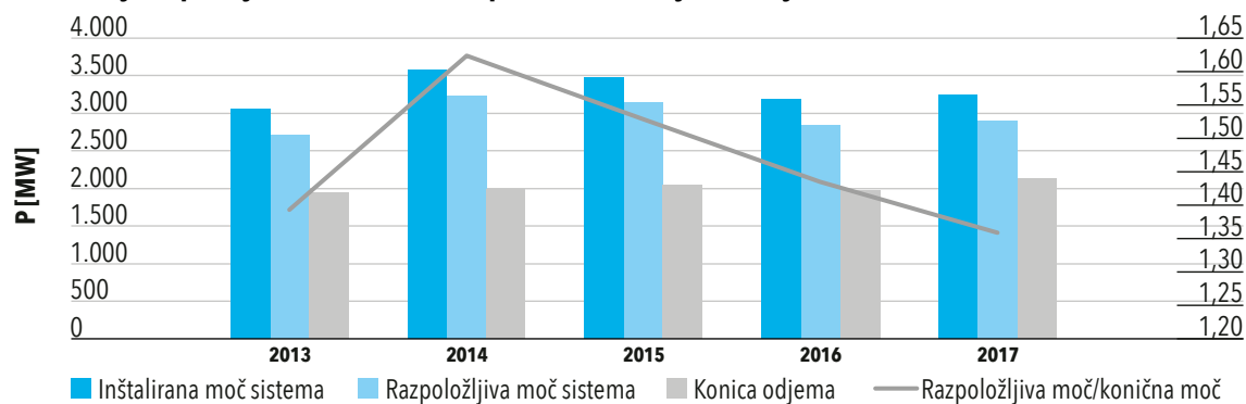
Slika 74: Inštalirane moči na pragu proizvodnih objektov, razpoložljive moči za slovenski trg in konična moč odjema ter razmerje razpoložljive in konične moči na prenosnem omrežju v obdobju 2013–2017
