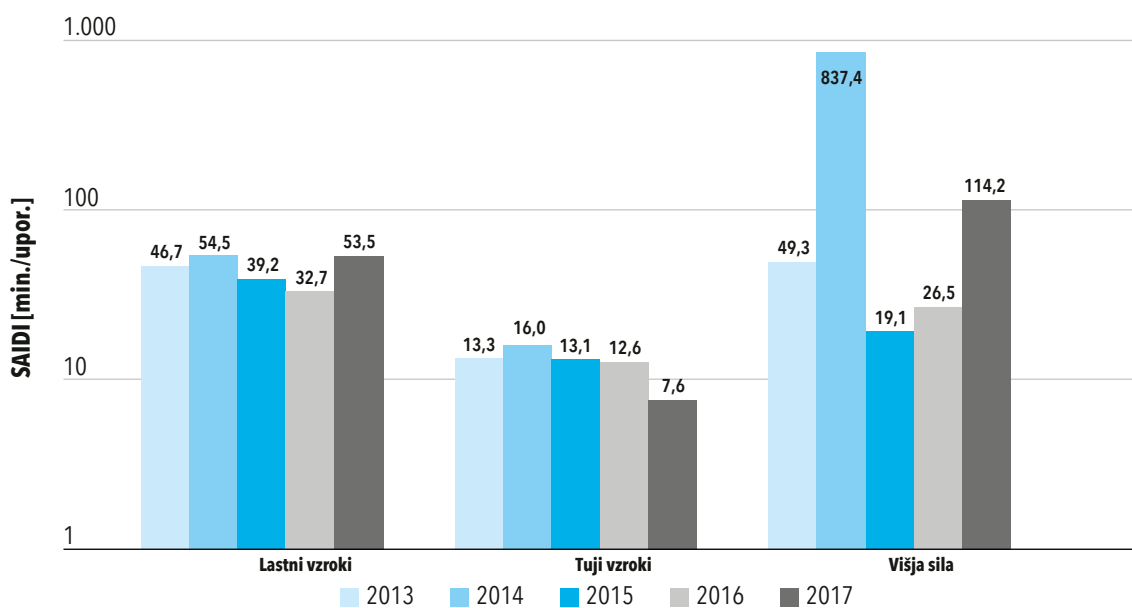
Slika 20: Parameter SAIDI za nenačrtovane dolgotrajne prekinitve, ločene po vzrokih, v obdobju 2013–2017
