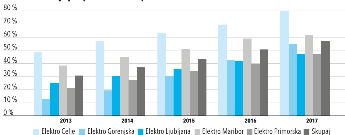
Slika 31: Trend uvajanja naprednih merilnih naprav
